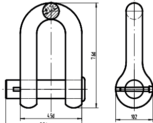
FORELOCK SHACKLE=FS
