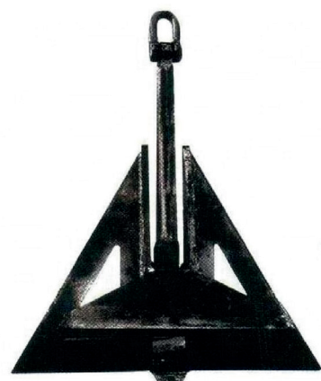
德尔塔锚 DELTA ANCHOR
