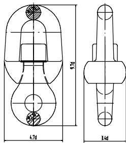
SWIVEL=SW
